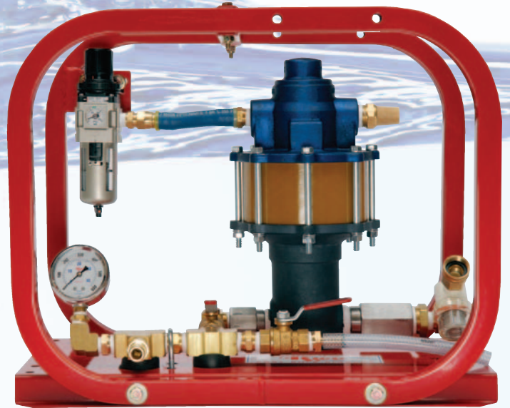
HP-3/500 • 500 PSI
